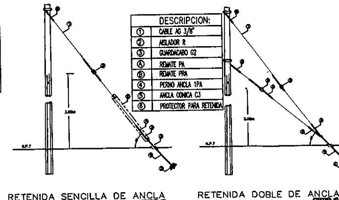
ESTRUCTURA TIPO TS20.
